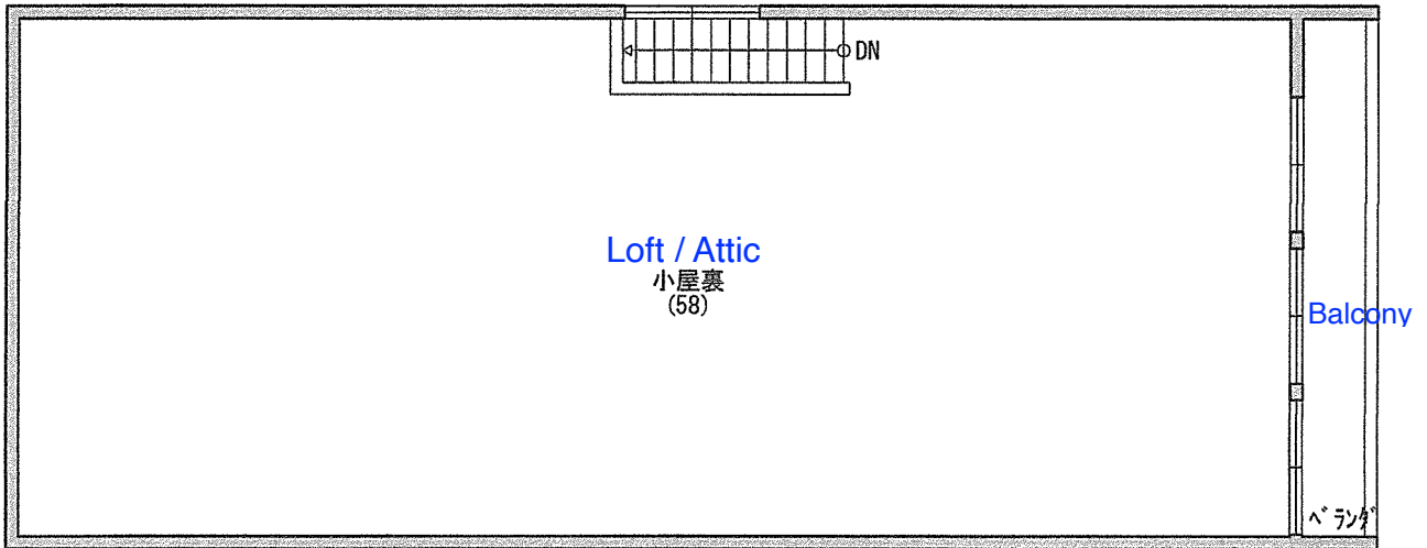
3rd Floor Plan 小屋裏平面図 S=1/100 (※29.7坪)
