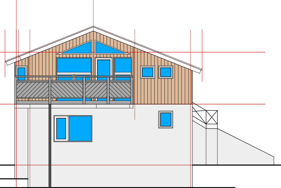
背面立面図
