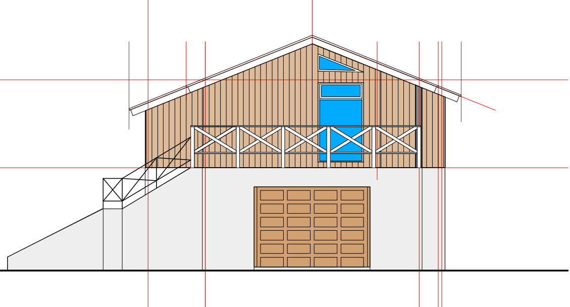
正面立面図
