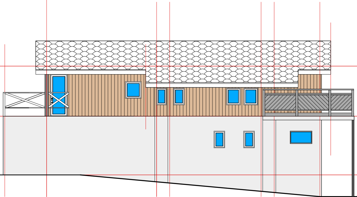
右側立面図
