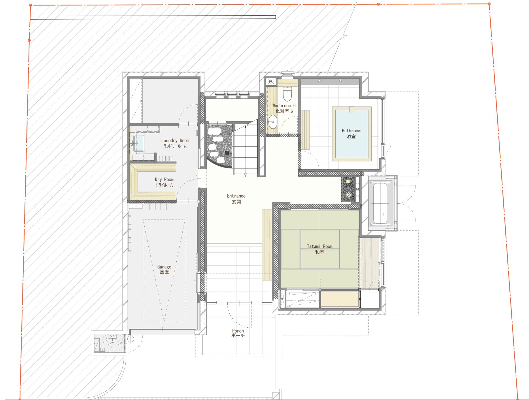
SOSEKI 礎石 1F
